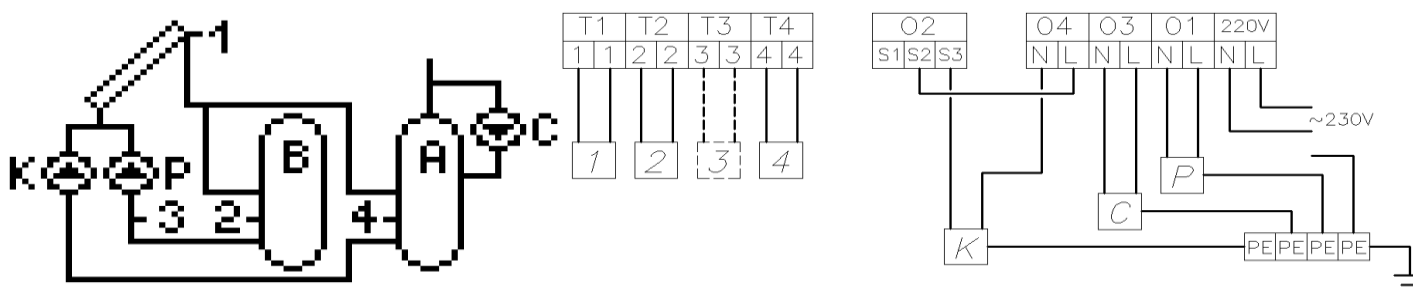
Rys. 21. Schemat ideowy oraz elektryczny instalacji układu nr 12.
