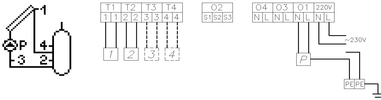
Rys. 10. Schemat ideowy oraz elektryczny instalacji nr 1.
