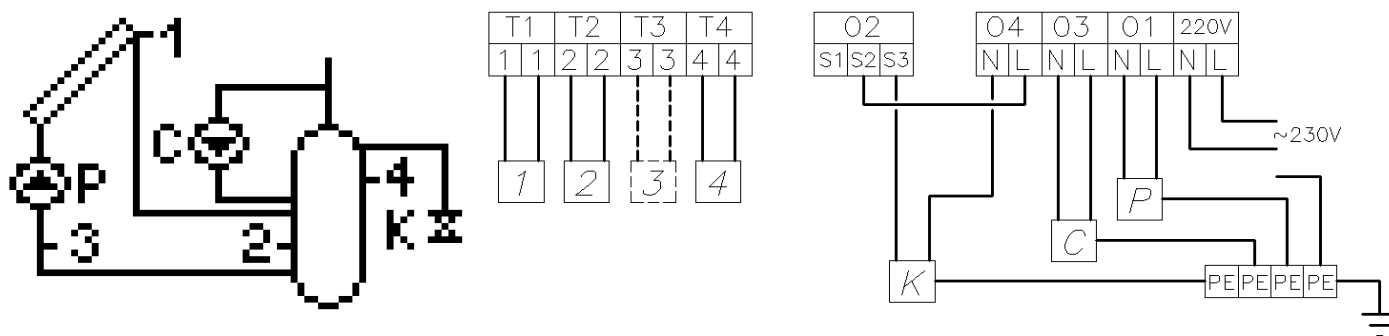
Rys. 26. Schemat ideowy oraz elektryczny instalacji układu nr 17.
