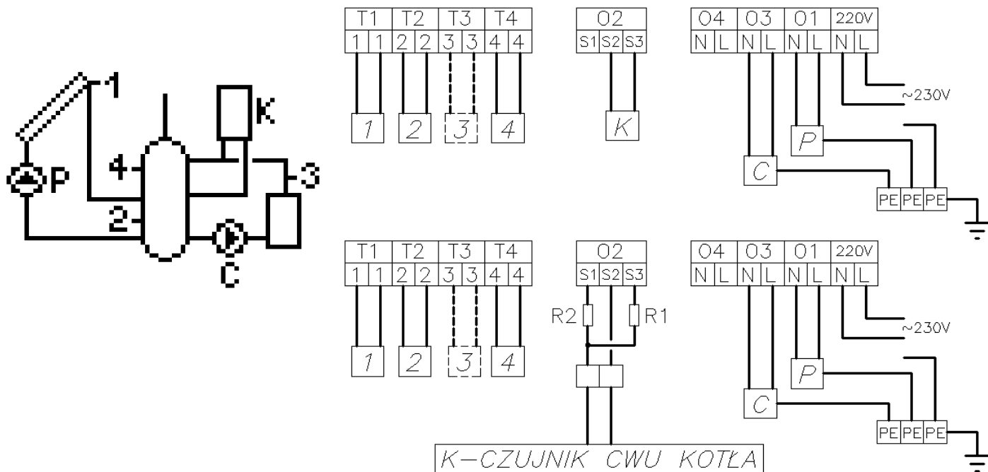
Rys. 23. Schemat ideowy oraz elektryczny instalacji układu nr 14.
