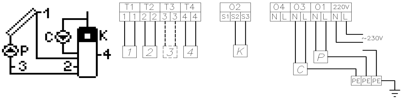
Rys. 14. Schemat ideowy oraz elektryczny instalacji nr 5.
