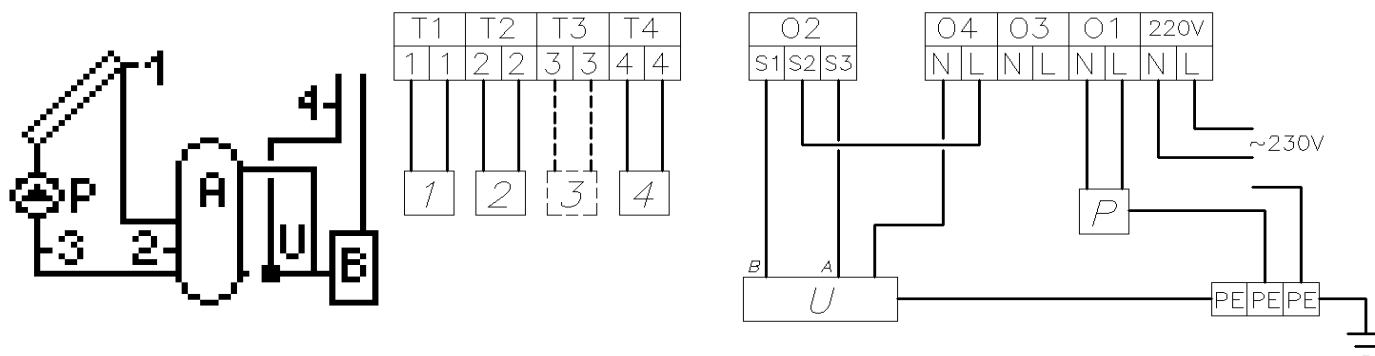
Rys. 22. Schemat ideowy oraz elektryczny instalacji układu nr 7.
