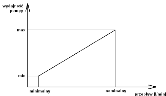
Rys. 9. Graficzne przedstawienie ustawionego przepływu.
