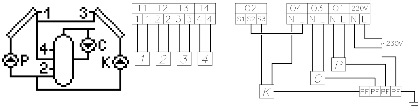
Rys. 24. Schemat ideowy oraz elektryczny instalacji układu nr 15.
