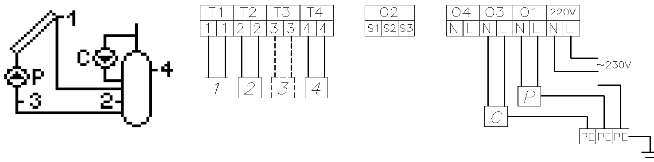
Rys. 11. Schemat ideowy oraz elektryczny instalacji nr 2.
