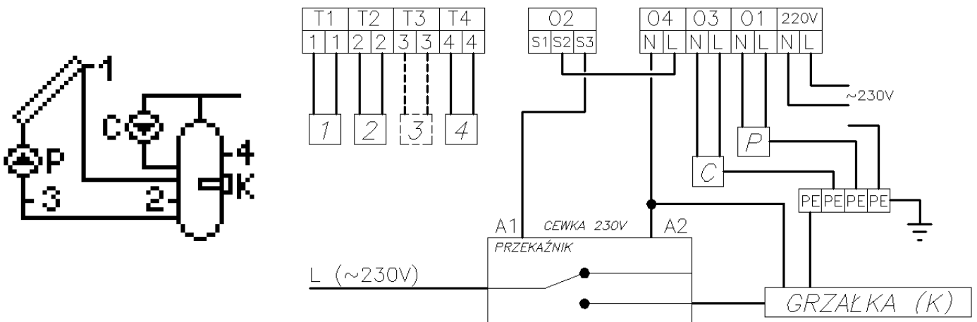
Rys. 13. Schemat ideowy oraz elektryczny instalacji nr 4.
